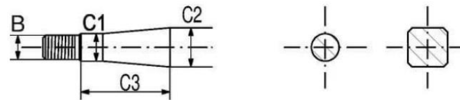
Рис. 2. Изогнутый зуб
